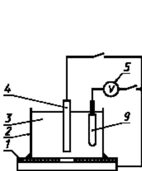
1 — пластина (карта) — испытуемый образец; 2 — труба из полиэтилена; 3 — электролит; 4 — магниевый анод; 5 — вольтметр; 9 — электрод сравнения
