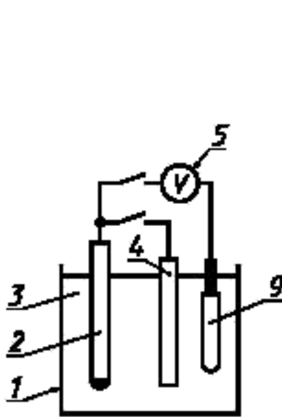
1 — емкость; 2 — испытуемый образец; 3 — электролит; 4 — магниевый анод; 5 — вольтметр; 9 — электрод сравнения
